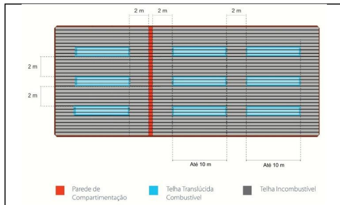
Figura 2: Afastamento de telhas combustíveis translúcidas
