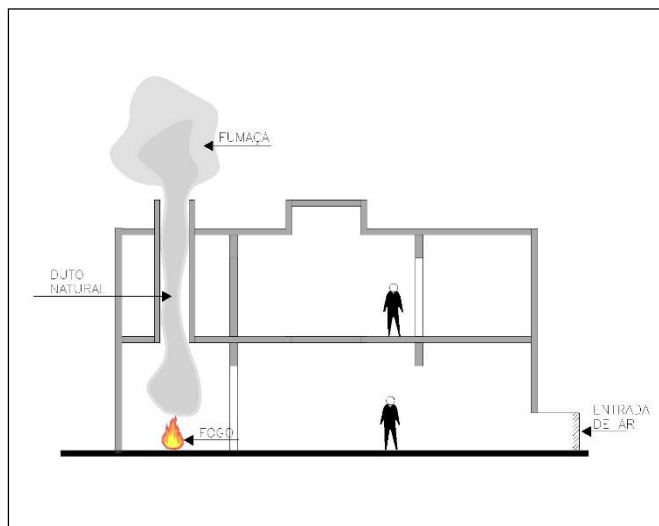
Figura 11: Exemplo de controle de fumaça por extração natural e entrada de ar natural, por meio de dutos
