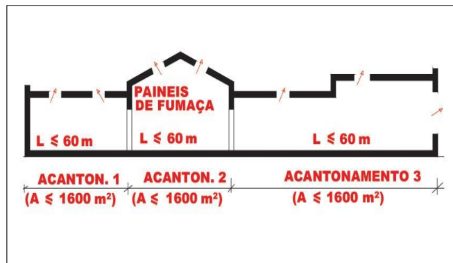
Figura 12: Divisão em áreas de acantonamento
