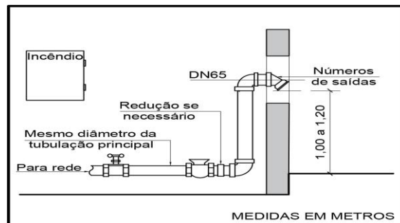
Figura 1: Dispositivo de recalque tipo coluna
