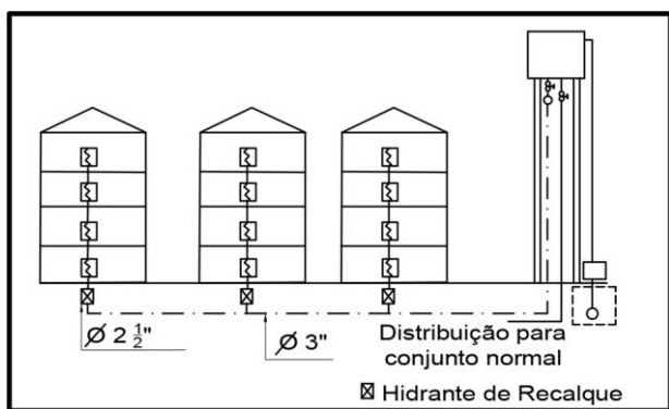
Figura 3: Esquema vertical
