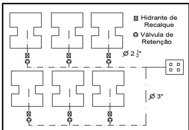
Figura 4: Esquema horizontal
