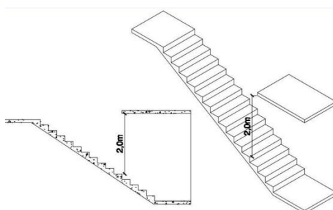
Figura 4 – Altura mínima de pé direito
