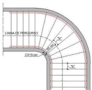
Figura 6 – Escada com lanço misto e degraus balanceados
