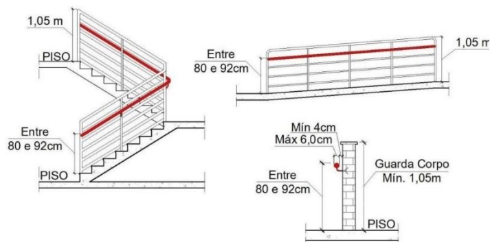
Figura 18 – Dimensões de guardas e corrimãos
