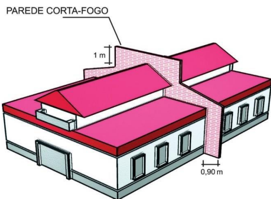
Figura 8: Parede corta-fogo
