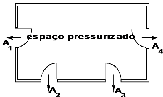
Figura 1: Trajetórias de escape do ar em paralelo
