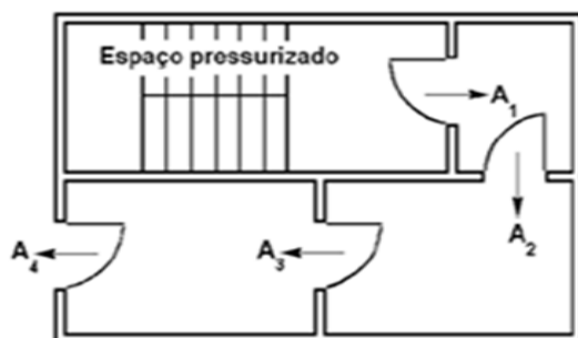
Figura 2: Trajetórias de escape do ar em série
